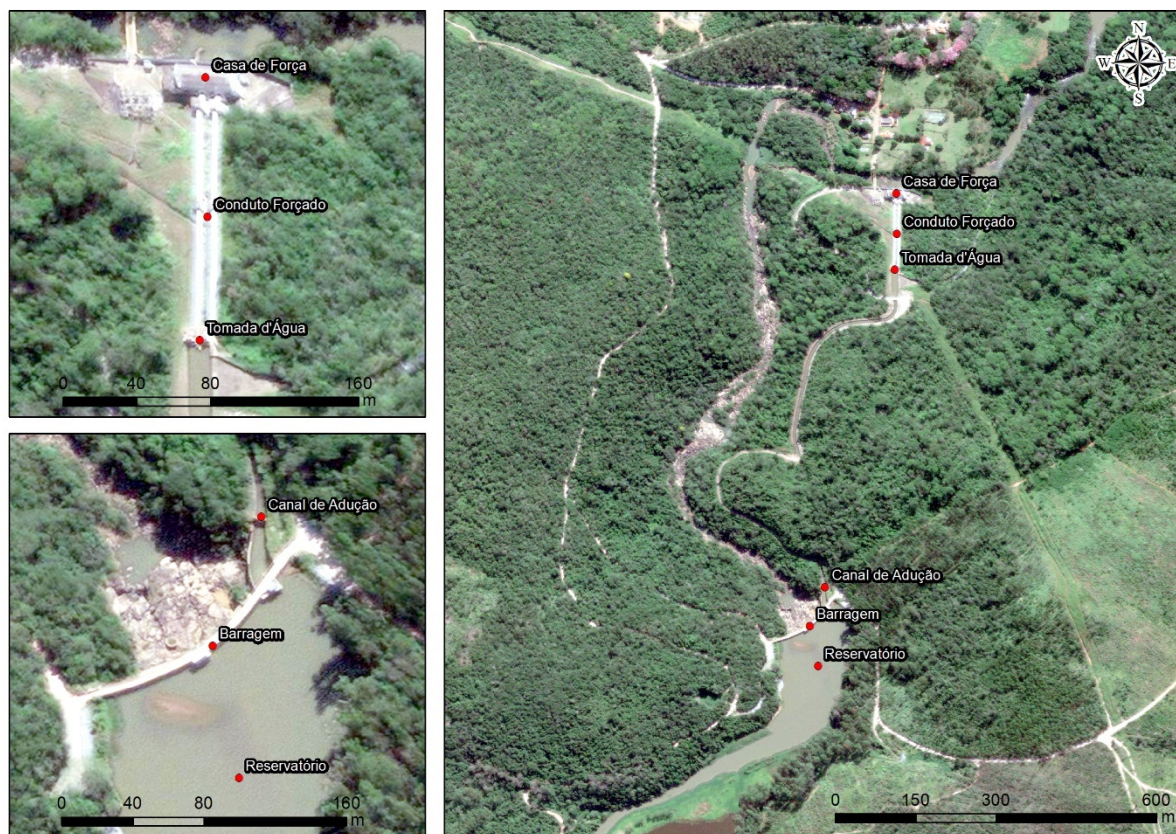
Figura 5 – Localização das estruturas na barragem da PCH Monte Alto
